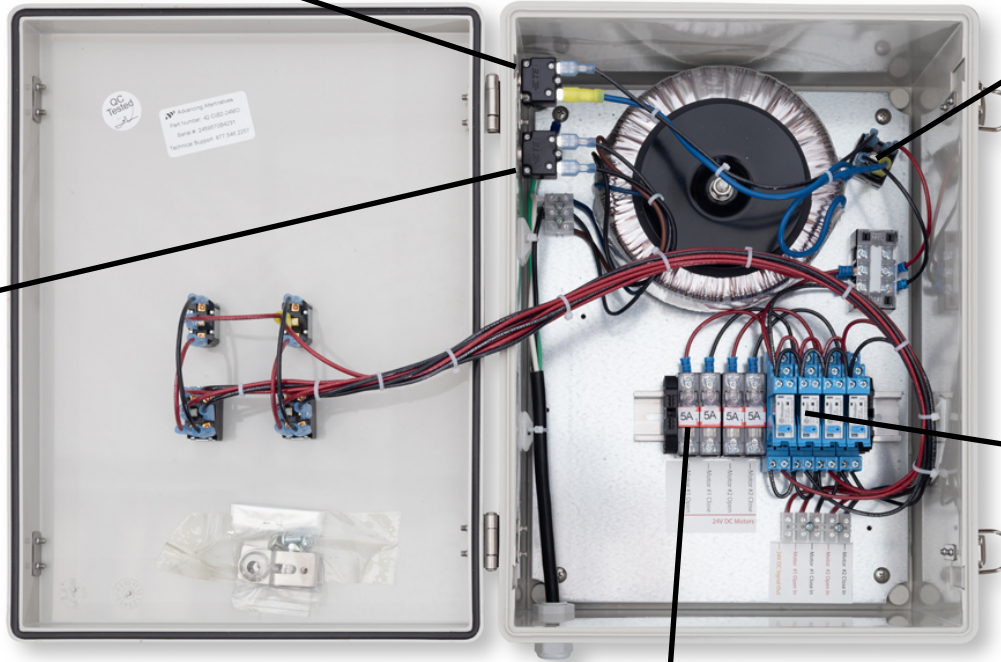
490-CBT-20A Circuit Breaker, Thermal, 20A
